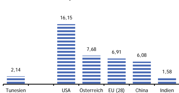
Kohlendioxidemissionen 2012 in Tonnen je Einwohner
